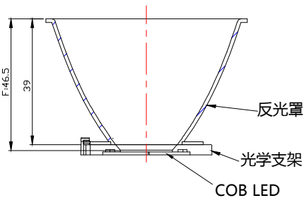
光学装配示意图
